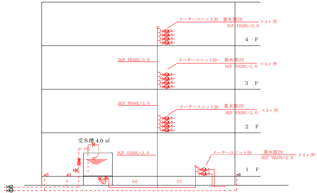
系統図
