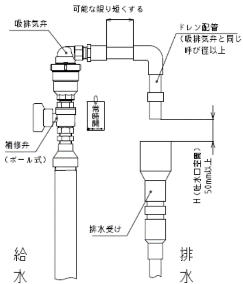
図3 吸排気弁の設置例
