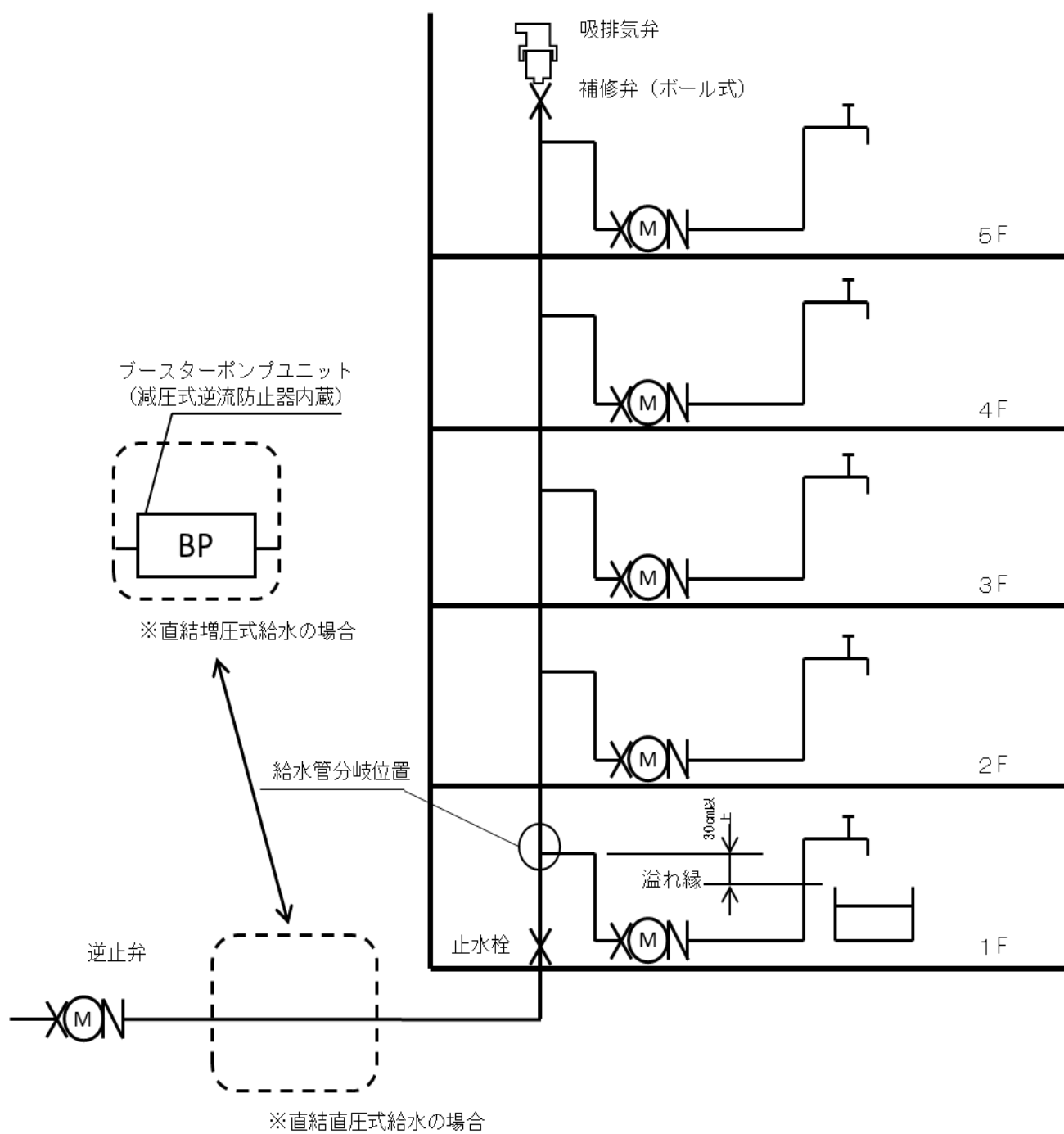
図2 逆流防止のイメージ図
