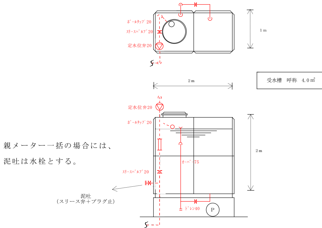
系統図
